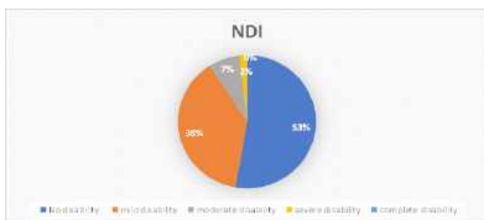
Figure 1: NDI.
